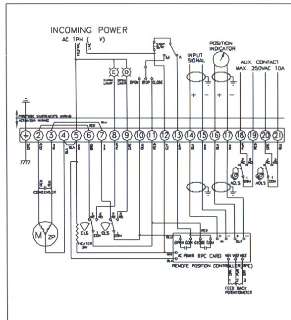
ATM0080(RPC)
