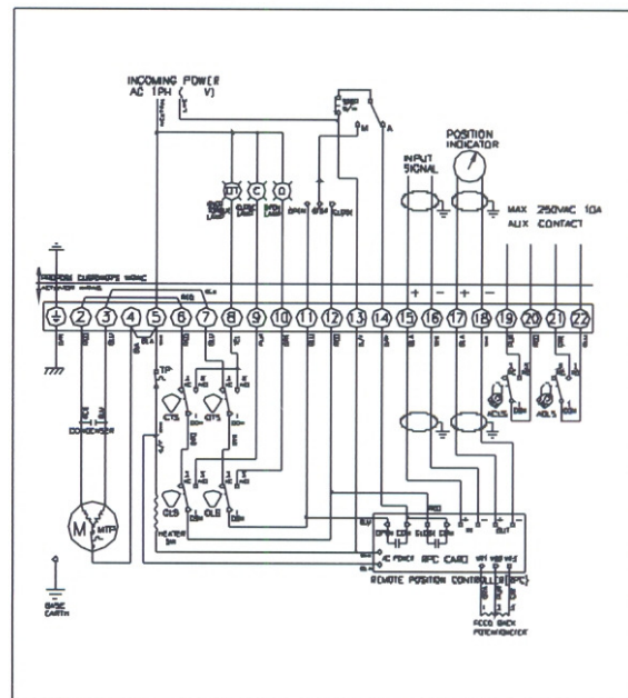
ATM0160~3000(RPC)
