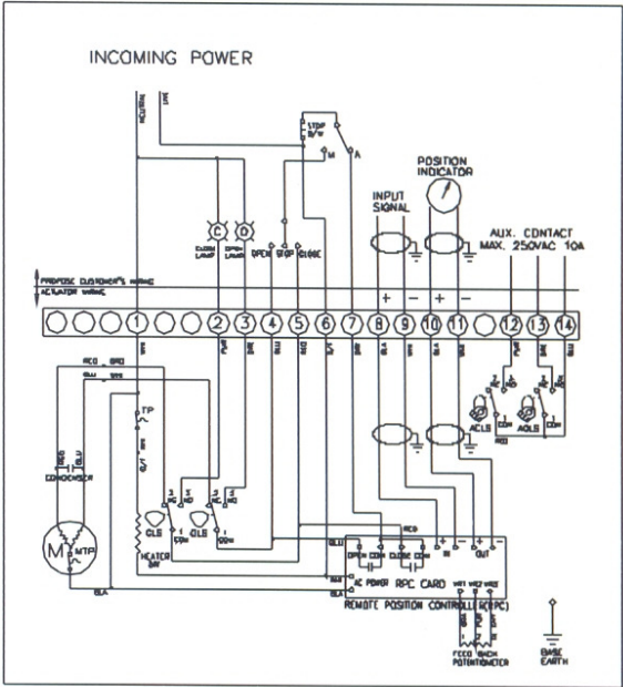
ATM0100(RPC)
